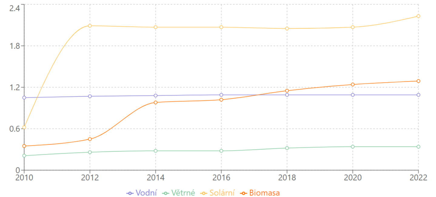
Vývoj instalovaného výkonu OZE v České republice (GW)
