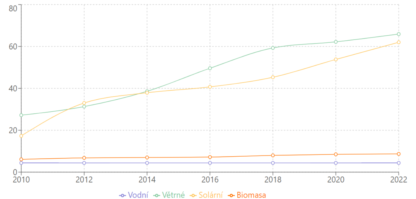
Vývoj instalovaného výkonu OZE v Německu (GW)
